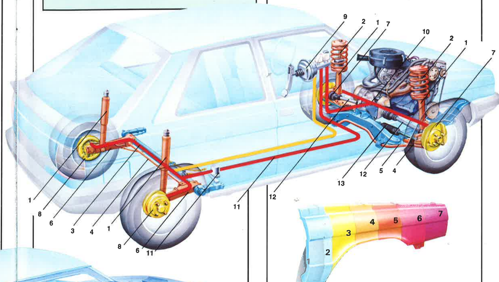
PROTECTION DE LA CARROSSERIE 1. Protection par écran polypropylène 2. Dégraissage chimique des tôles 3. Phosphatation au zinc 4. Passivation chromique
