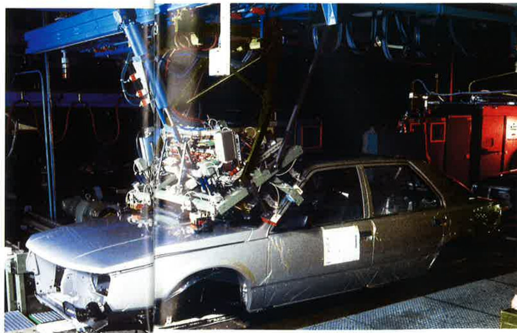
Opération de pose par robot d'un pare-brise sur une Renault 25
