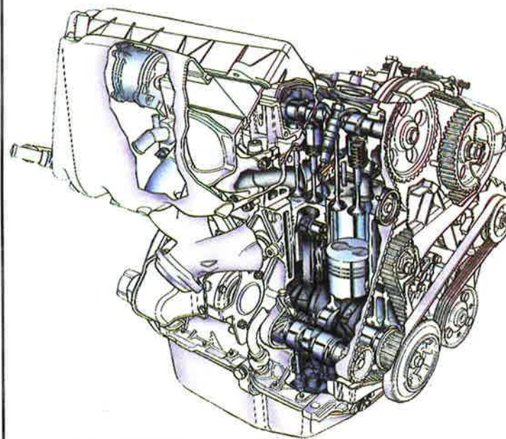
MOTEUR 1595 CM 3 DIESEL
